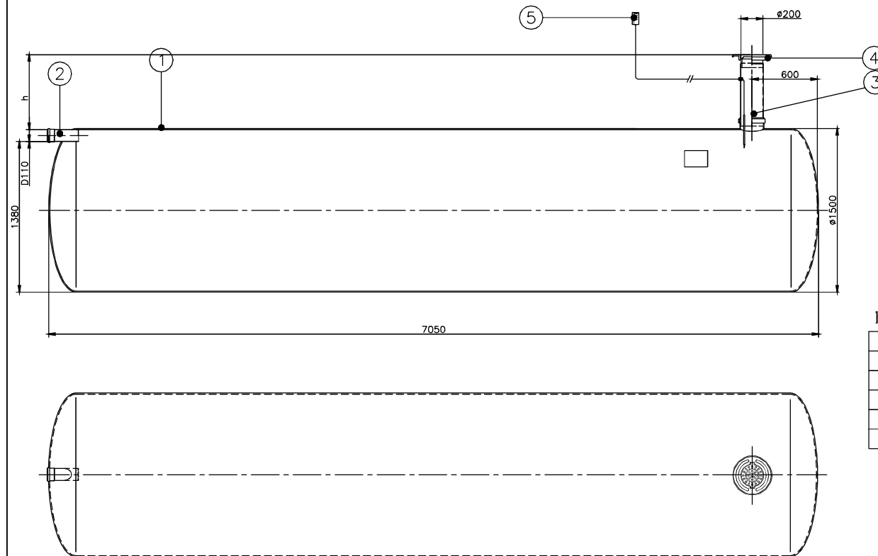
Joonis: Reoveemahuti 12m 3
