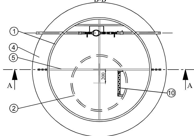
PEALTVAADE B-B
