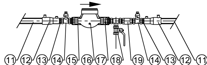
VEEMÕÖDUSÕLME TÜÜPSKEEM
